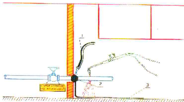
Rys.2. Spawane przewody, części maszyn i urządzeń oraz elementy konstrukcji budowlanych stykające się z materiałami palnymi lub przebiegające w pobliżu nich należy skutecznie chłodzić: 1-przewód doprowadzających wodę, 2-zwoje sznura z włókna szklanego, 3-koc szklany.
