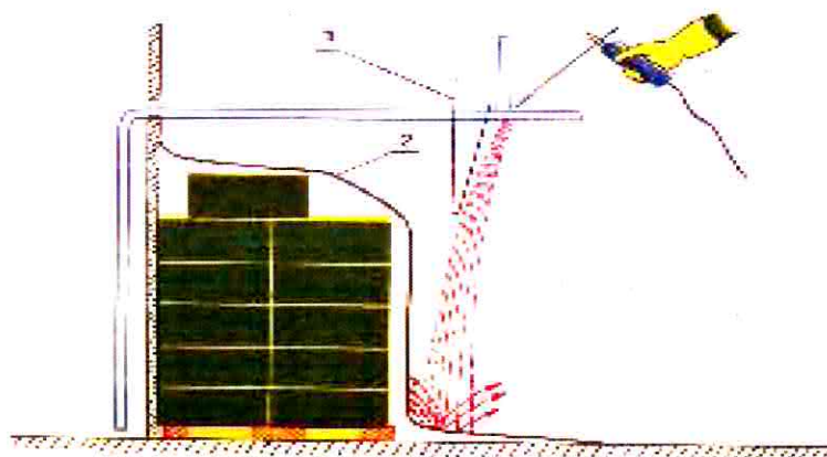
Rys.1. Materiały palne, których nie można odsunąć poza zasięg rozprysków spawalniczych osłaniamy w sposób gwarantujący bezpieczeństwo: 1-ekran z blachy, 2-koc z tworzywa szklanego.
