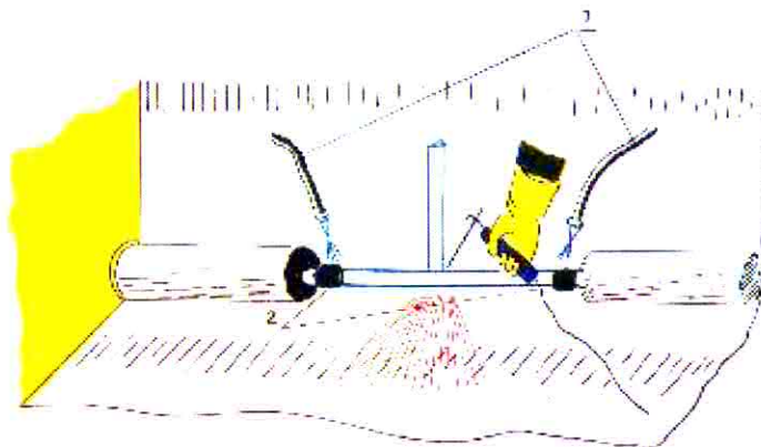
Rys.4. Z izolowanych rurociągów, na których prowadzi się prace spawalnicze, należy usunąć izolację cieplną na odcinku gwarantującym bezpieczeństwo, a w razie potrzeby chłodzić skutecznie: 1-przewody doprowadzające wodę, 2-zwoje sznura z włókna szklanego.
