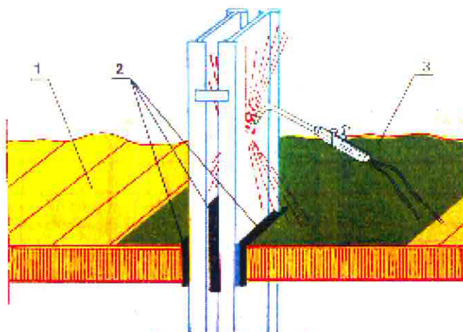
Rys.6. Sposób prawidłowego zabezpieczenia spawania metalowego elementu konstrukcji przechodzącego przez drewniany strop: 1-drewniany strop, 2-szczeliwo z włókna szklanego, 3-koc szklany.
